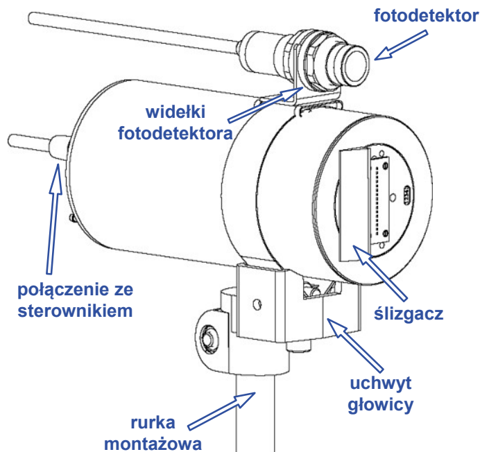
Rys. 2.3.2.1. Mocowanie standardowego uchwytu głowicy elektromagnetycznej
