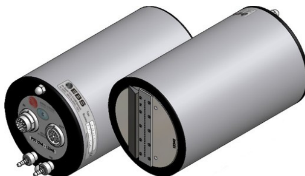
Głowica elektromagnetyczna 25 do 32 dysz
